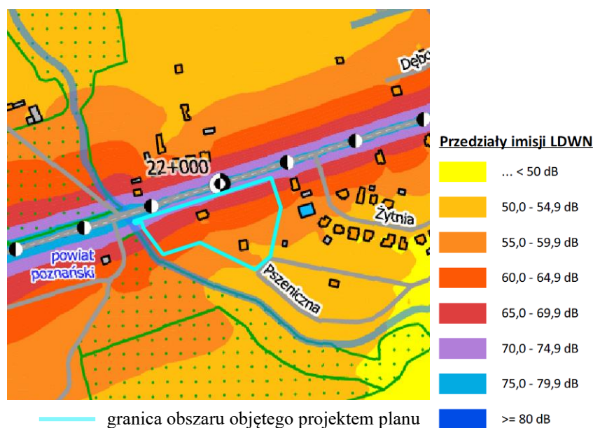
Ryc. 8. Mapa imisyjna dla odcinka drogi wojewódzkiej nr 307 - wskaźnik L_{DWN} [dB]
