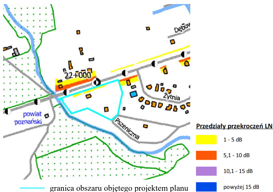
Ryc. 10. Mapa terenów zagrożonych hałasem dla odcinka drogi wojewódzkiej nr 307 - wskaźnik L_{DWN} [dB]
