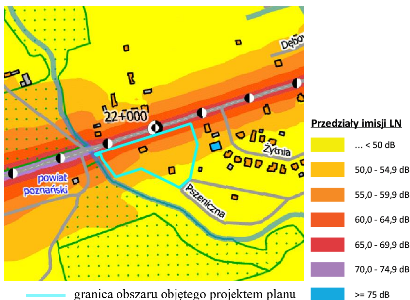
Ryc. 9. Mapa imisyjna dla odcinka drogi wojewódzkiej nr 307 - wskaźnik L_N [dB]
