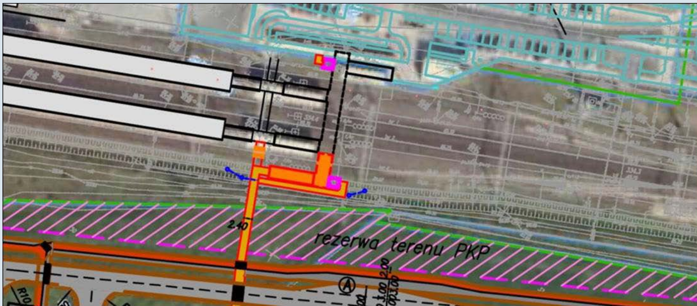
Szkic sytuacyjny planowanego przedłużenia przejścia podziemnego w kierunku południowym pod linią kolejową E20 w rejonie stacji Buk
